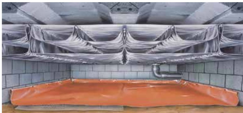
Dwarsdoorsnede thermokussens
