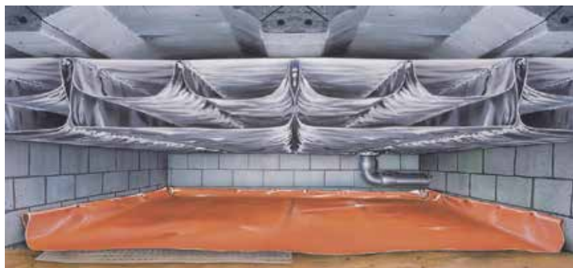
Dwarsdoorsnede thermokussens
